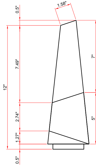
LEFT
