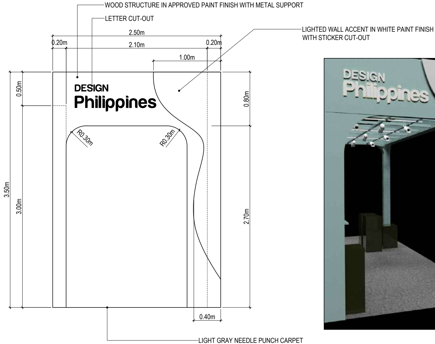
ELEVATION A
