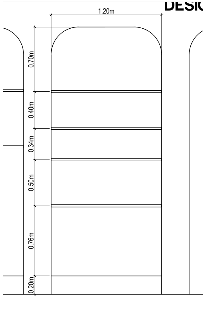
ELEVATION
