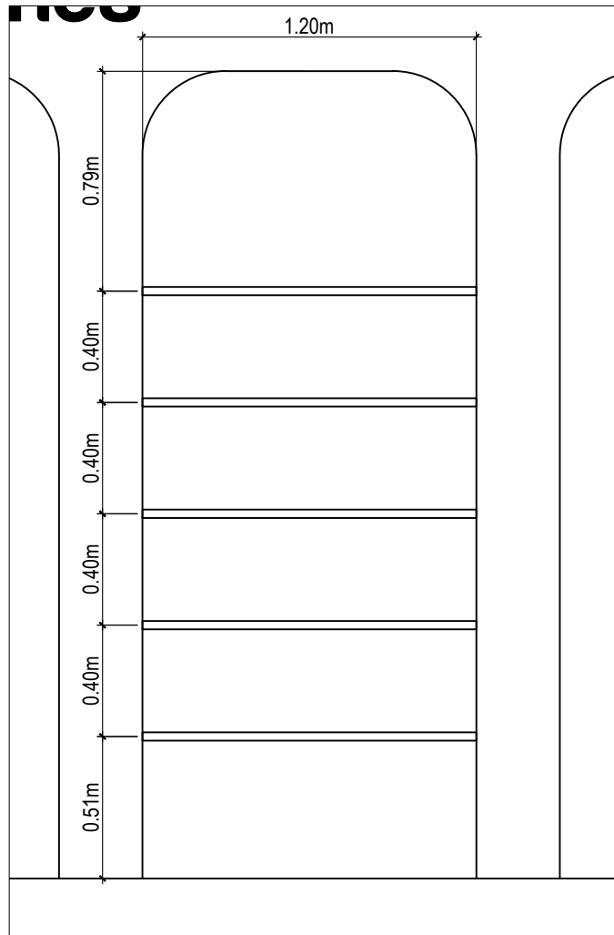
ELEVATION
